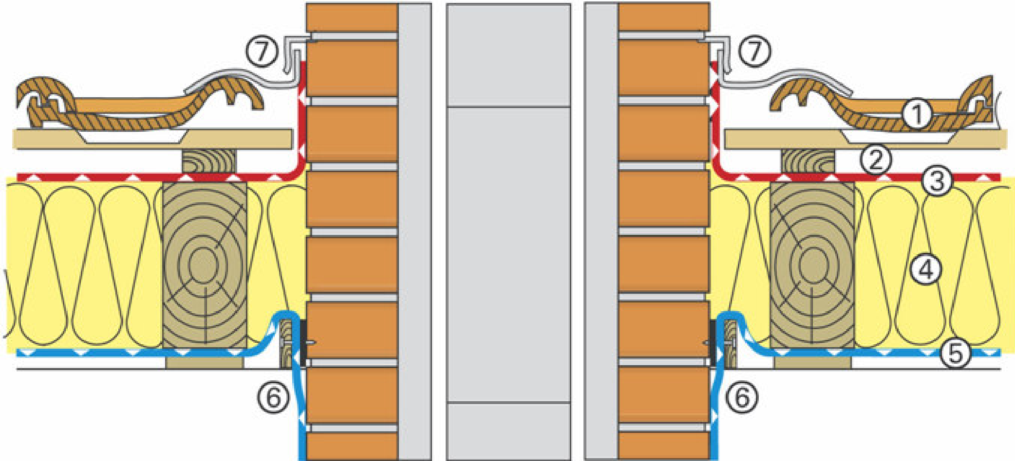
Kaminanschluss Bild 2
